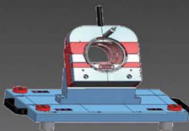
汽车出风口总成检具
